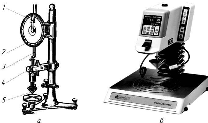
Рис. 6.1. Приборы для определения пенетрации: a – пенетромтр ПН-1ЖВ; б – пенетромтр K95590 (Koechler Instrument); 1 – стрелка циферблата; 2 – циферблат; 3 – кремальера; 4 – пусковая кнопка; 5 – конус
