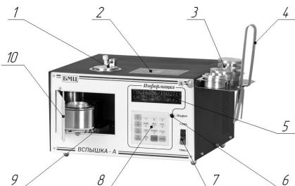
Рис. 5.1. Автоматический регистратор температуры вспышки нефтепродуктов «Вспышка-А»:
