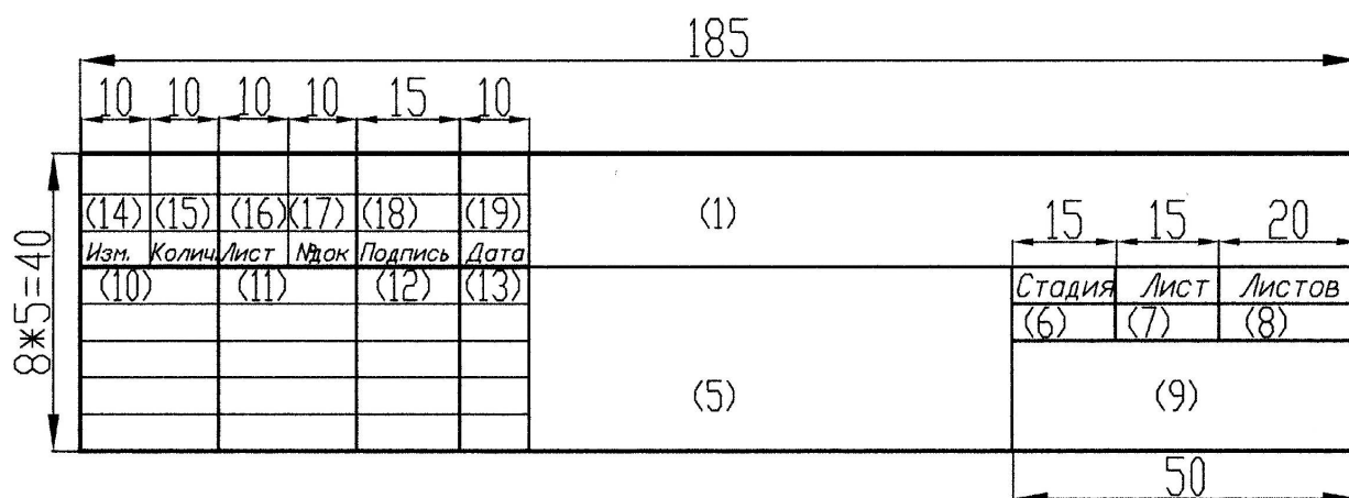
Рисунок 10 – Форма основной надписи, которая применяется для листа РПЗ, с которой начинается изложение текстовой части записки (обычно лист «Оглавление»)
