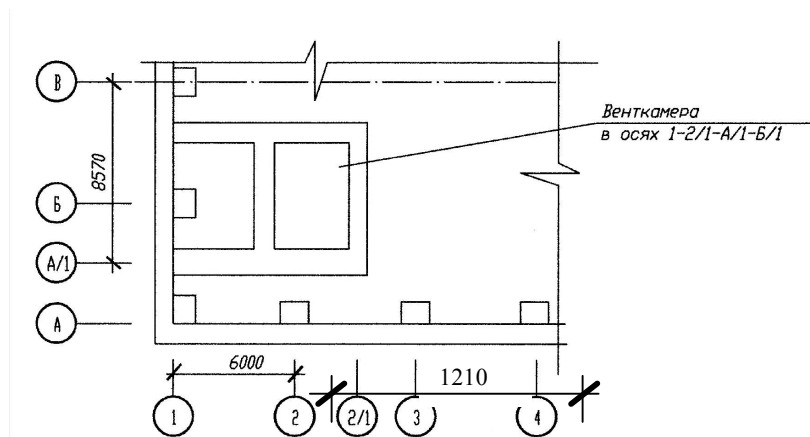
Рисунок 13 – Оформление обозначений осей
