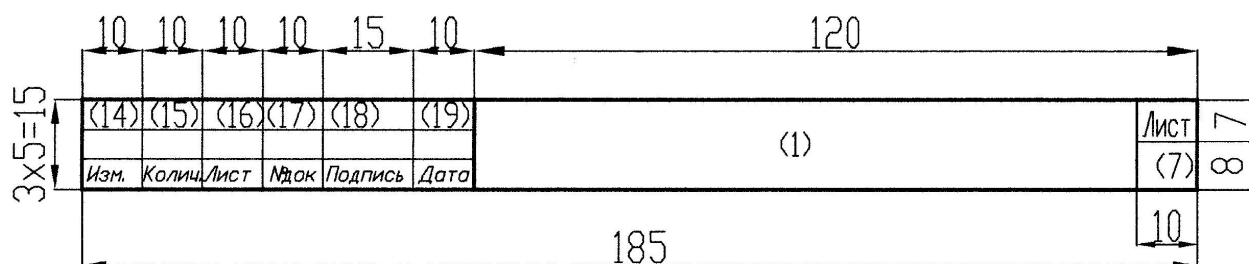
Рисунок 11 – Форма основной надписи, которая применяется для последующих листов РПЗ и чертежей
