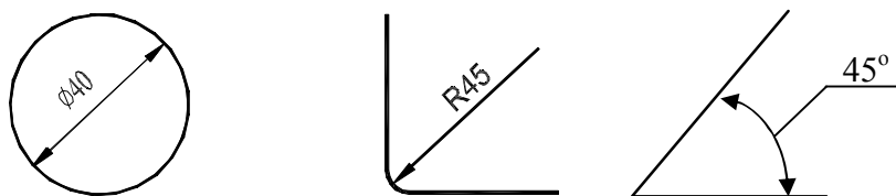
Рисунок 14 – Оформление нанесения размеров
