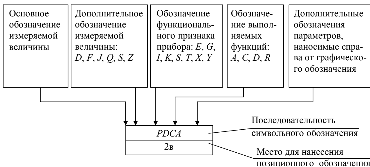
Рисунок 18 – Принцип построения условного обозначения прибора
