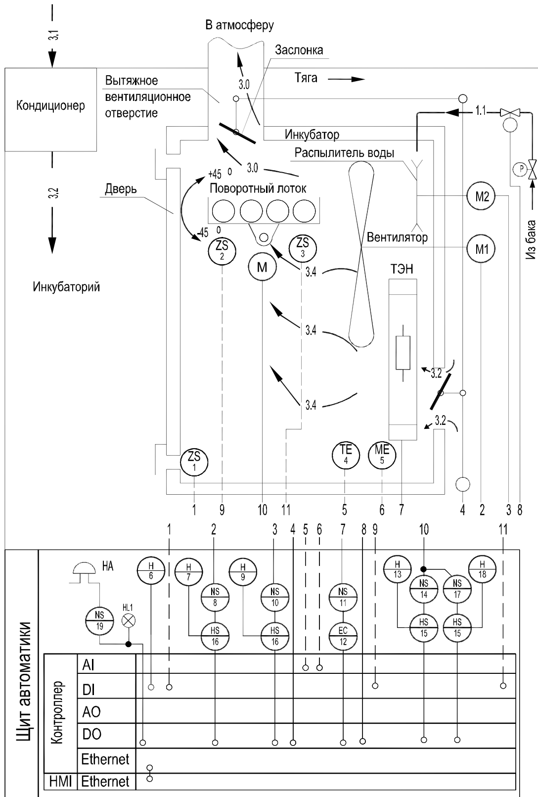
Рисунок 17 – Схема автоматизации инкубатора
