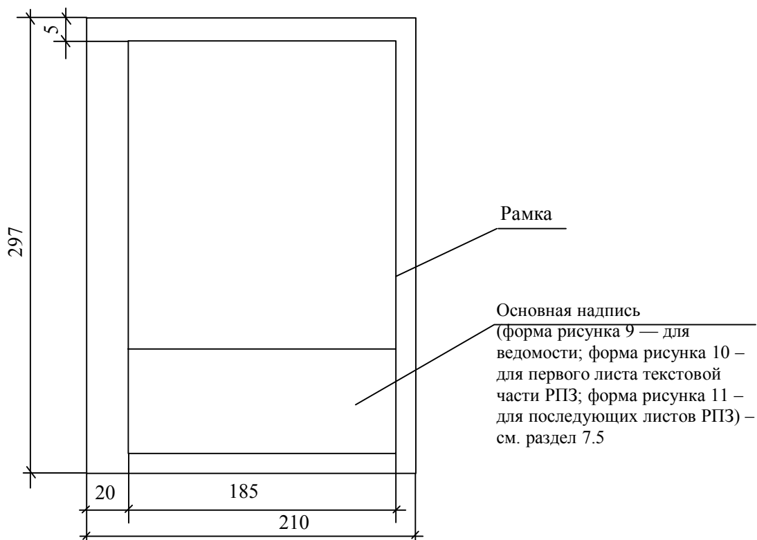
Рисунок 1 – Компоновка и размеры листа текстовой части РПЗ
