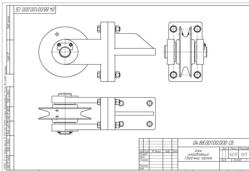
Рис. 7.2. Вставка трех стандартных видов с 3D-модели
