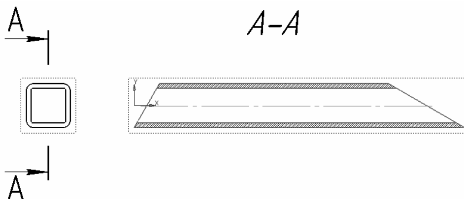
Рис. 12.3. Разрез детали «Раскос»
